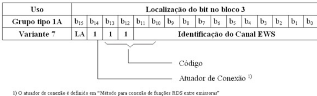
Figura 34: Estrutura da variante 7 do bloco 3 do grupo 1 A (identificação de uma emissora que transporta informações EWS)
